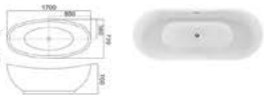
C-3251-15 Size:720x1500x680/mm C-3251-17 Size:720x1700x700/mm
